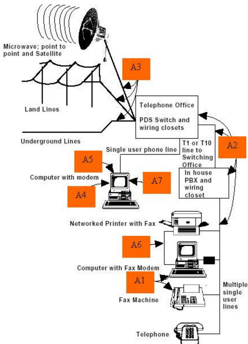
Figura 4 Posibile amenințări (notate A1 – A7) la adresa faxurilor, de-a lungul rețelei de linii telefonice comutate
